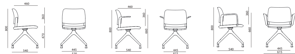
Trespolo su piedini Trestle base with gliders Base quadripie con regaton
