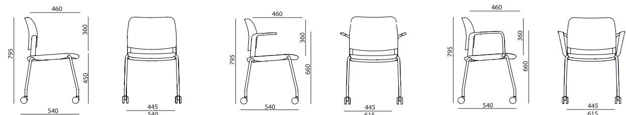
Quattro gambe su ruote Four legs frame with castors Quatro patas con ruedas
