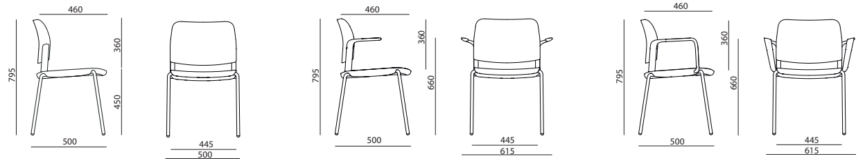
Quattro gambe Four legs frame Quatro patas
