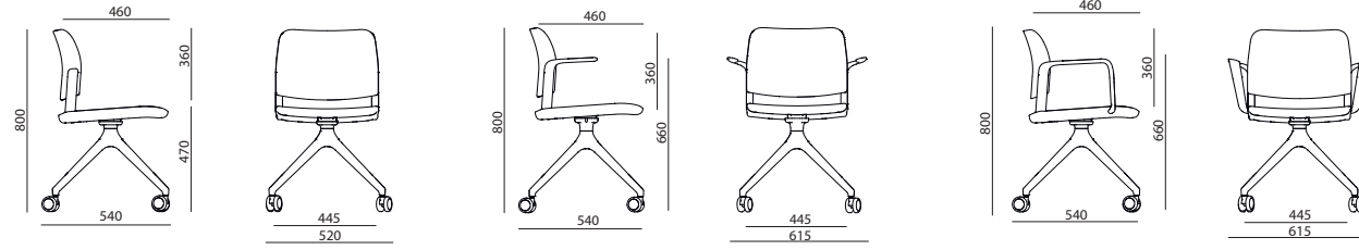
Trespolo su ruote Trestle base with castors Base quadripie con ruedas
