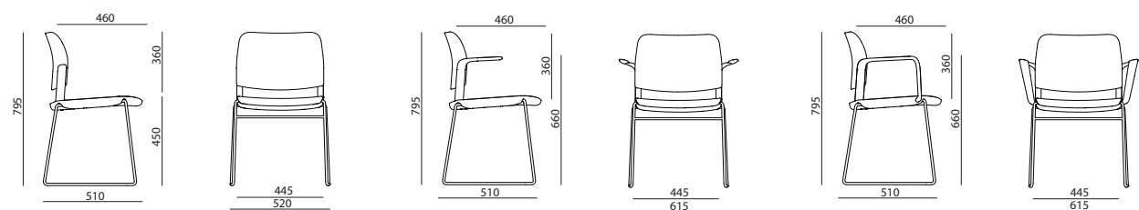
Fusto tondino Rod frame without armrests Estructura de varilla sin reposabrazos
