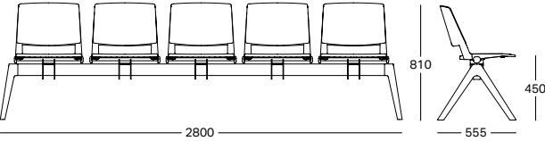
Panca 5 posti con gamba GP04 5 seater bench with GP04 leg Banco de 5 plazas con pata GP04
