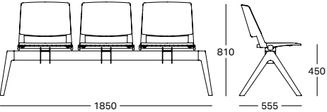
Panca 3 posti con gamba GP04 3 seater bench with GP04 leg Banco de 3 plazas con pata GP04
