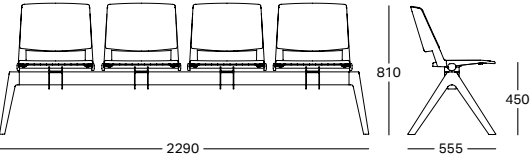
Panca 4 posti con gamba GP04 4 seater bench with GP04 leg Banco de 4 plazas con pata GP04
