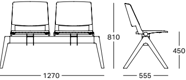
Panca 2 posti con gamba GP04 2 seater bench with GP04 leg Banco de 2 plazas con pata GP04
