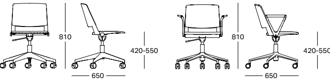
Base girevole R42N R42N swivel base Base giratoria R42N Base girevole R35 R35 swivel base Base giratoria R35
